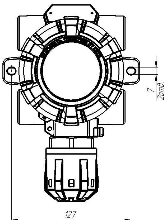
Рисунок 5 – Монтажные размеры
