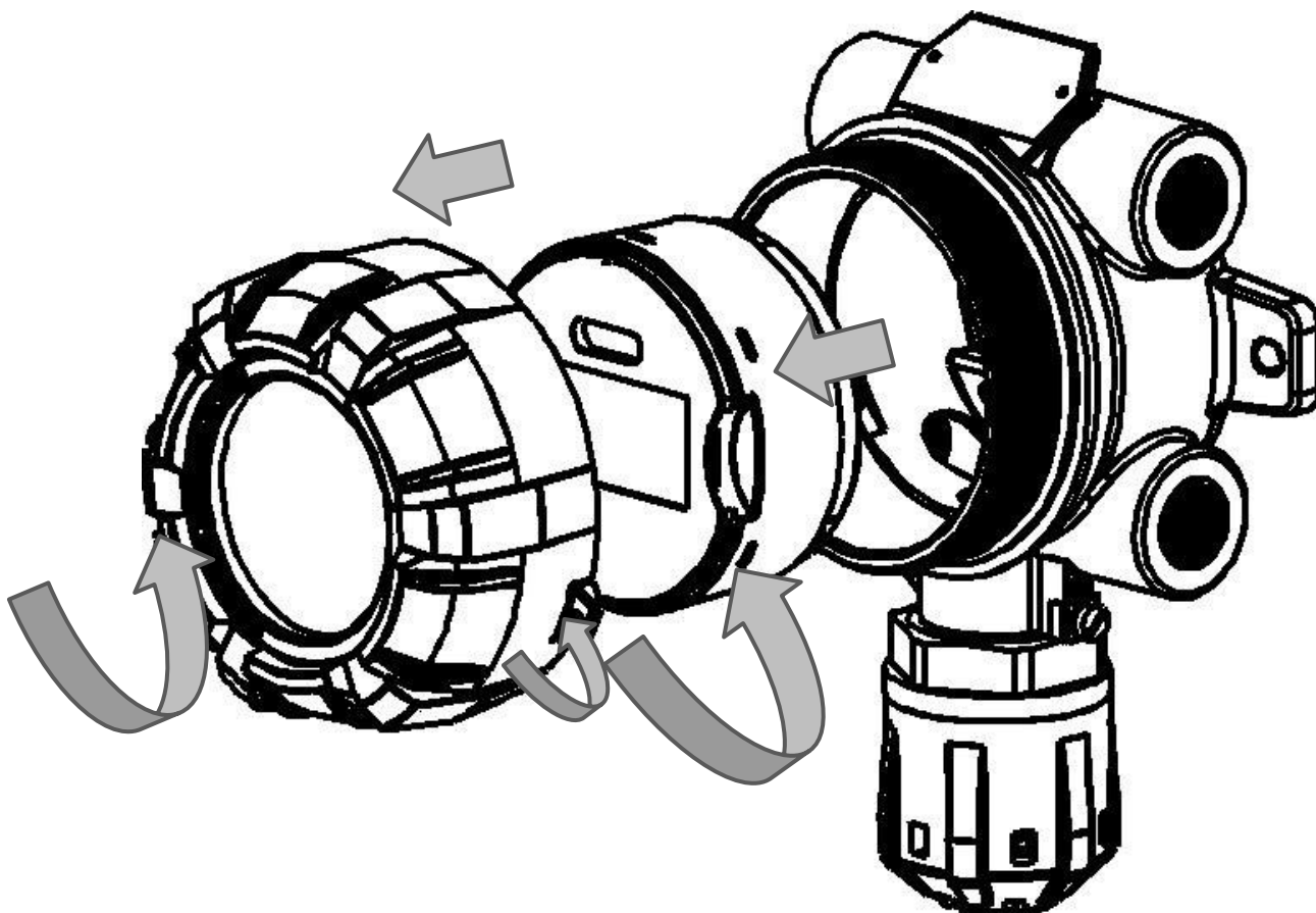
Рисунок 14 - Схема разбора газоанализатора
