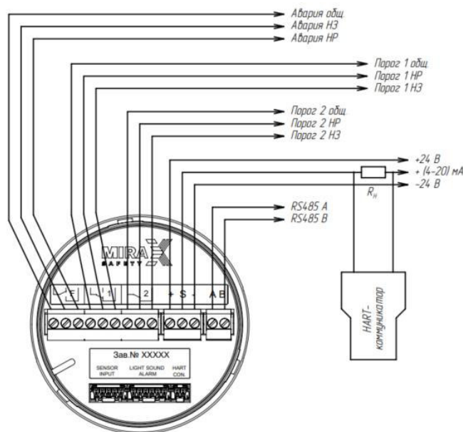
Рисунок 12 – Схема подключения газоанализатора AXIOM
