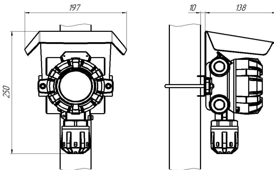
Рисунок 10 - Монтаж козырька газоанализатора
