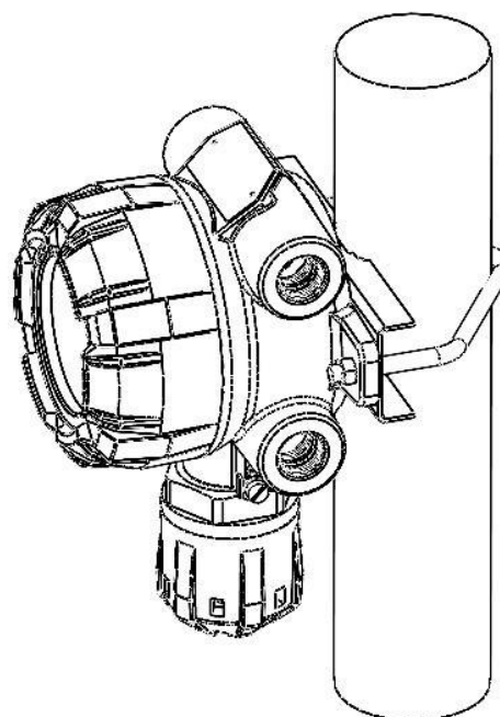
Рисунок 8 – Вид газоанализатора, установленного на трубу
