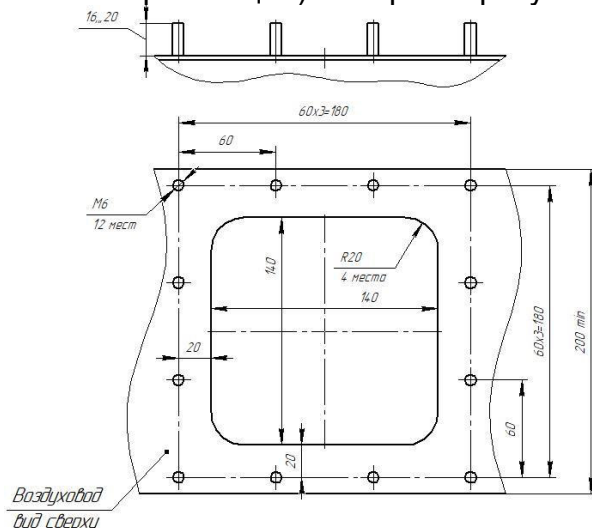
Рисунок 9 – Место для установки комплекта
